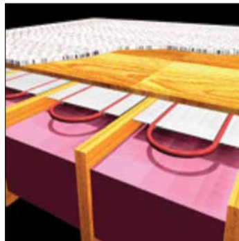
Systèmes avec plaquettes de transfert de chaleur sous ou sur le plancher
